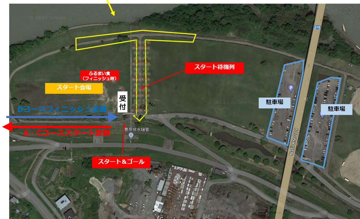
会場拡大図
